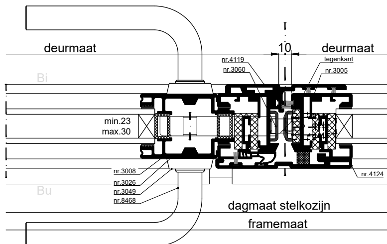
HORIZONTALE DOORSNEDE type XIS-1A/E
