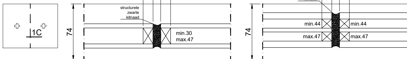
structurele glasverbinding zonder afdekprofiel
