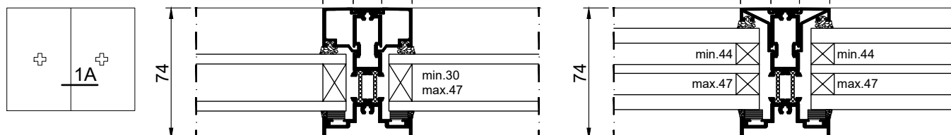
verticale tussenstijl
