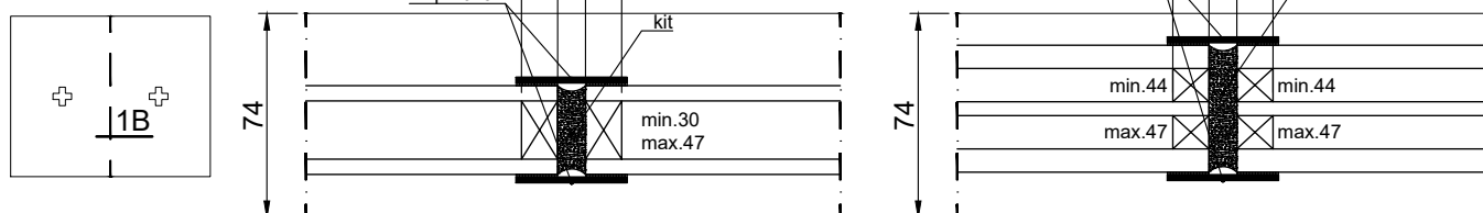
structurele glasverbinding incl. afdekprofiel
