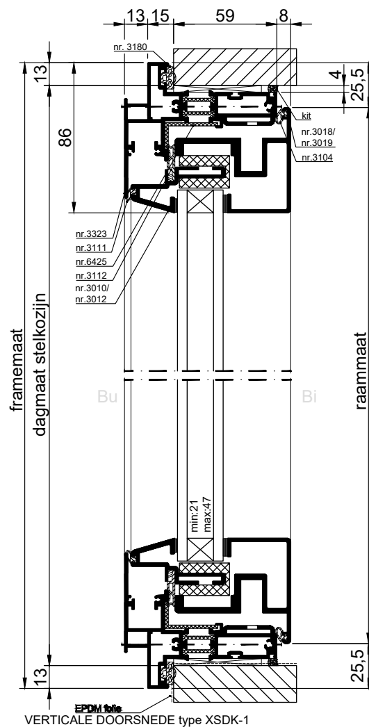
EPDM tafe VERTICALE DOORSNEDE type XSDK-1
