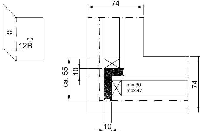
structurele glasverbinding zonder afdekprofiel
