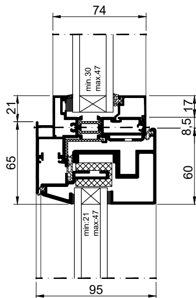
horizontale tussenstijl
