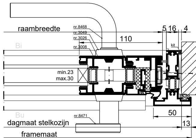
HORIZONTALE DOORSNEDE type XID-1B/C/D/F
