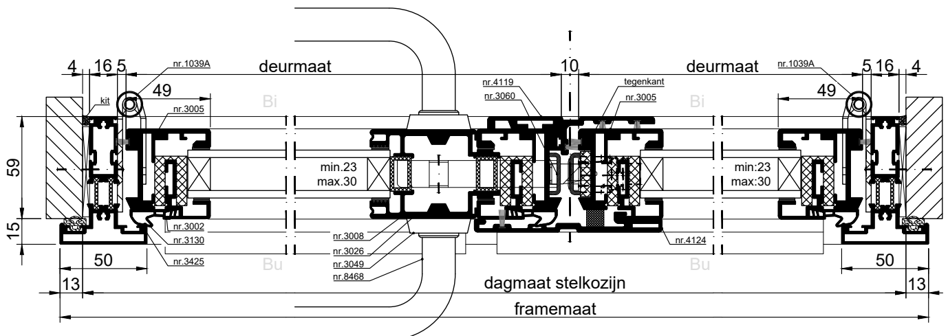
HORIZONTALE DOORSNEDE type XIS-1A
