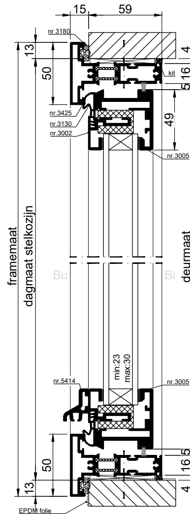
VERTICALE DOORSNEDE type XIS-1A
