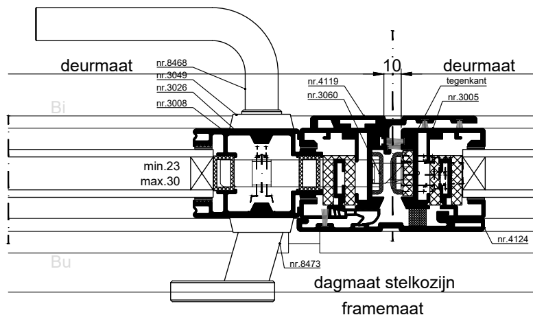
HORIZONTALE DOORSNEDE type XIS-1B/C/D/F
