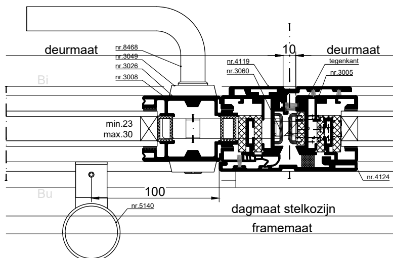
HORIZONTALE DOORSNEDE type XIS-1G/H
