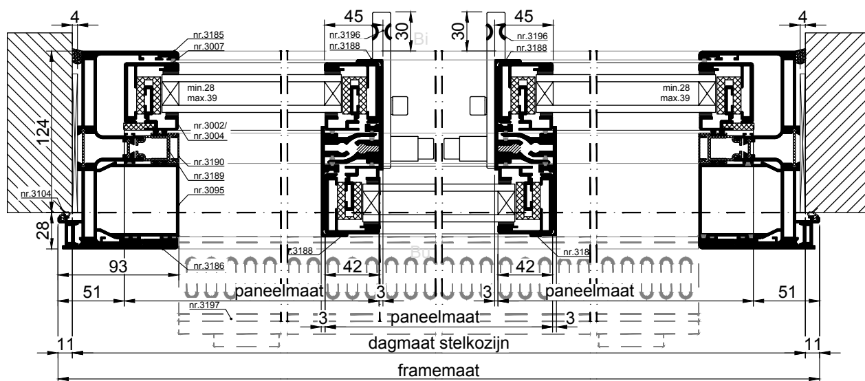
HORIZONTALE DOORSNEDE type XHS-9D
