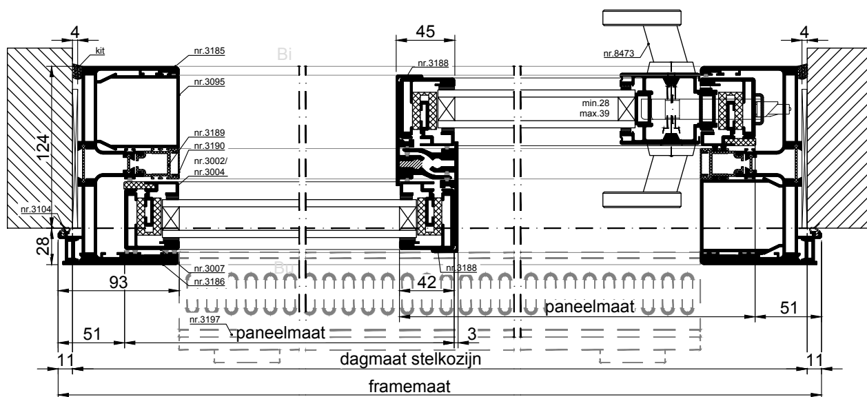
HORIZONTALE DOORSNEDE type XHS-10A
