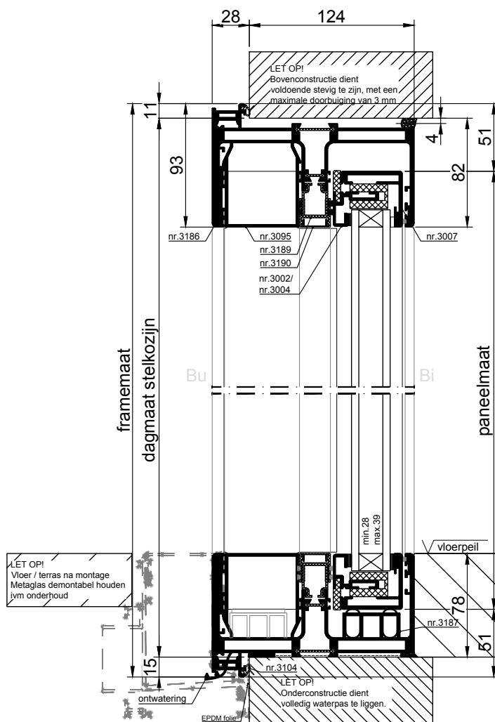
VERTICALE DOORSNEDE type XHS-9D
