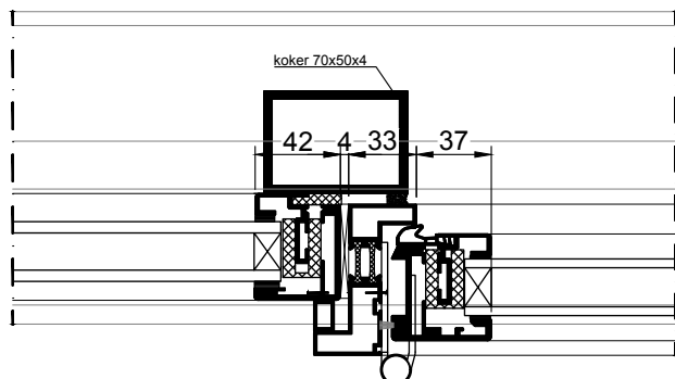
verticale tussenstijl vast paneel met deur
