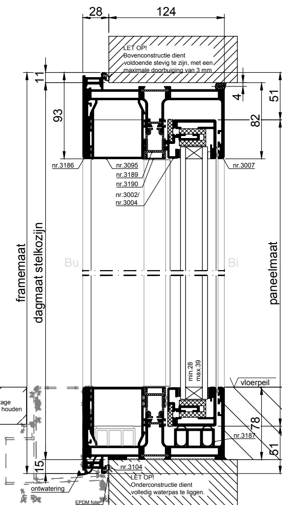
VERTICALE DOORSNEDE type XHS-10E
