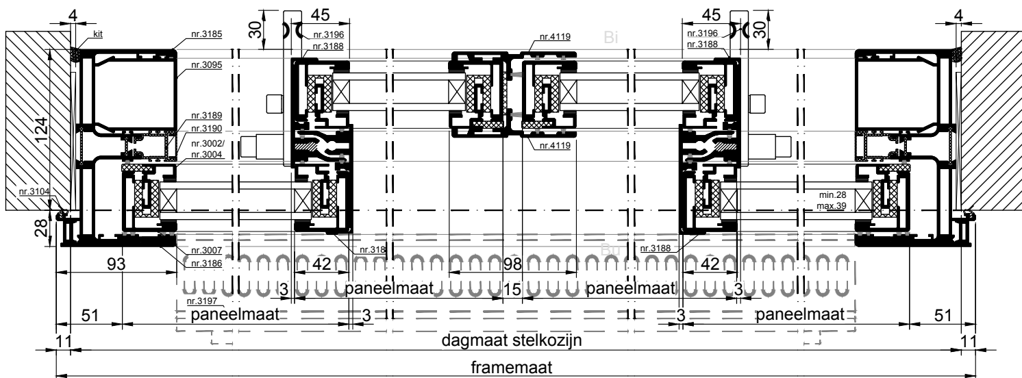
HORIZONTALE DOORSNEDE type XHS-9E
