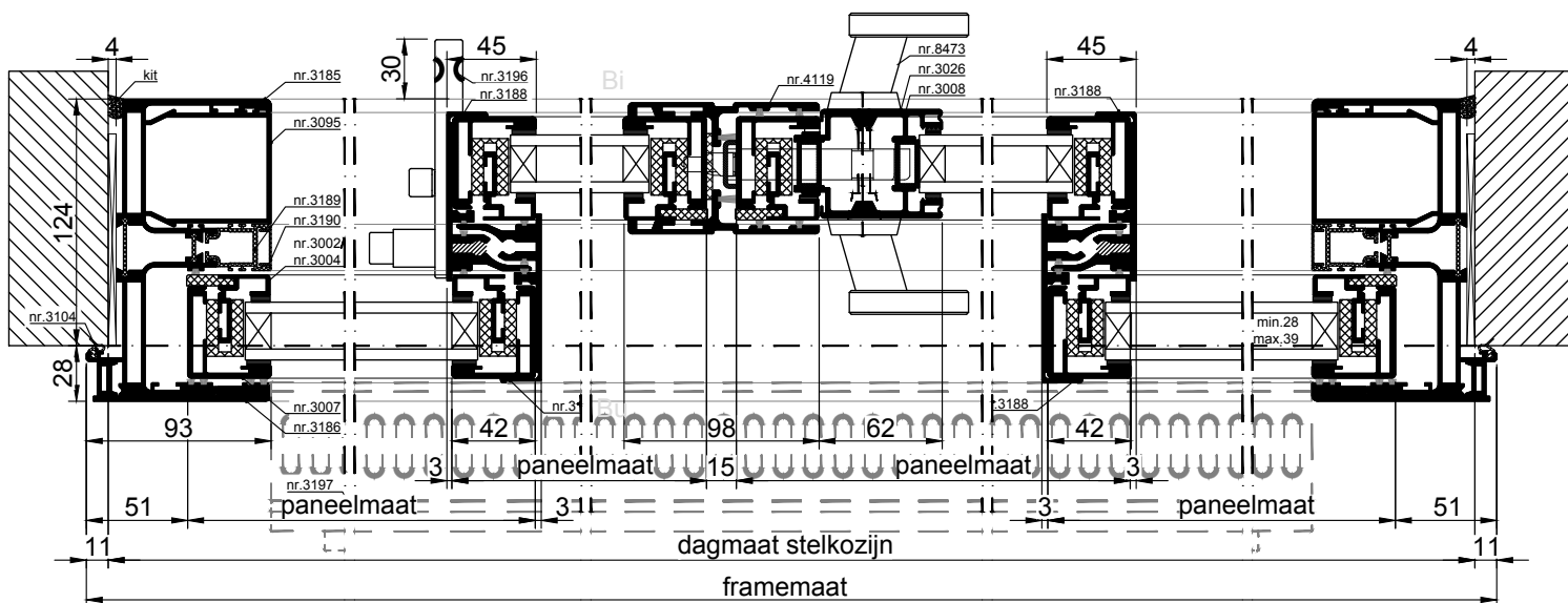
HORIZONTALE DOORSNEDE type XHS-10E
