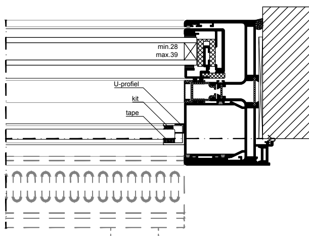
horizontaal onderprofiel met doorvalbeveiliging
