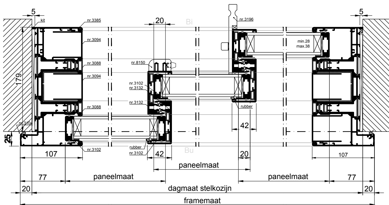
HORIZONTALE DOORSNEDE type XHS-30C
