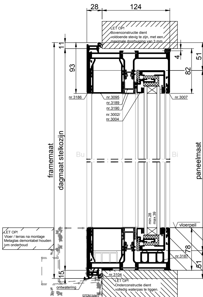
VERTICALE DOORSNEDE type XHS-9C
