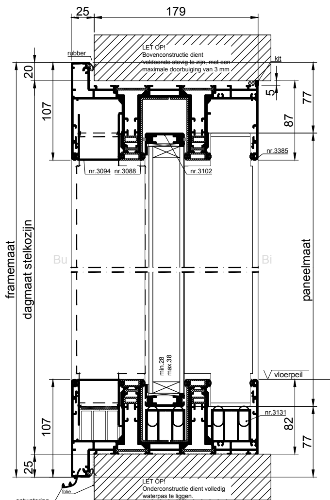
VERTICALE DOORSNEDE type XHS-30C
