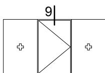
horizontaal bovenprofiel met deur
