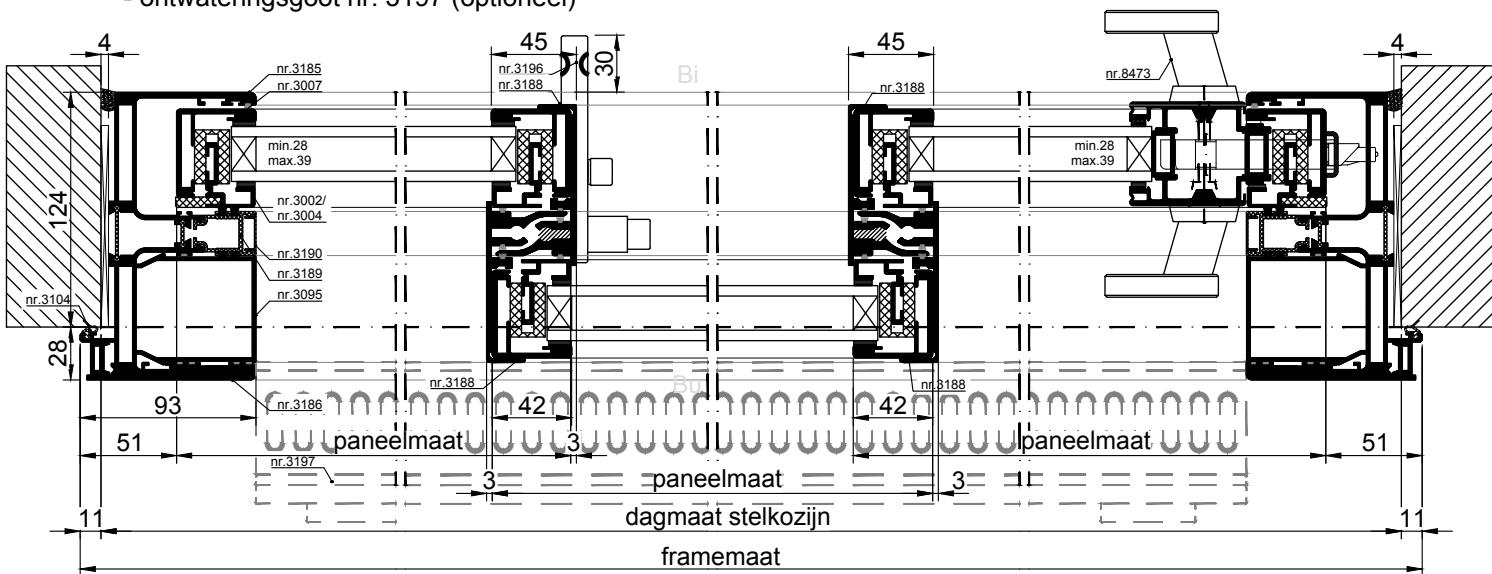
HORIZONTALE DOORSNEDE type XHS-10D
