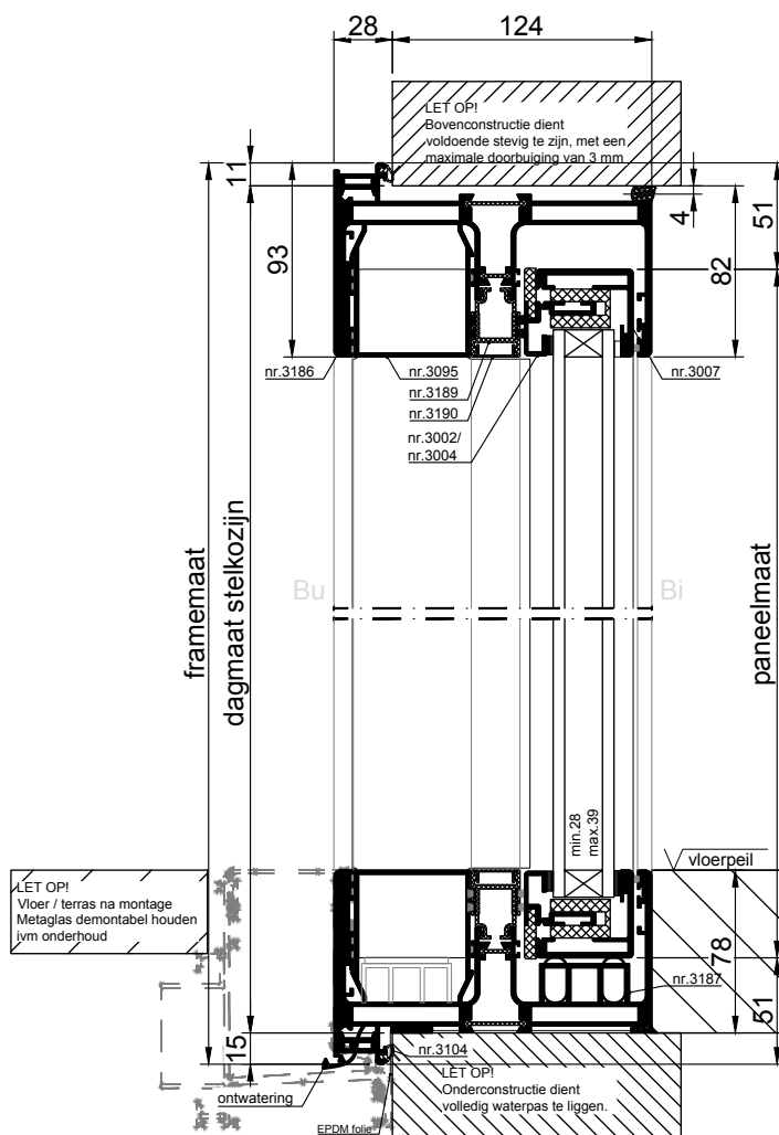
VERTICALE DOORSNEDE type XHS-9A
