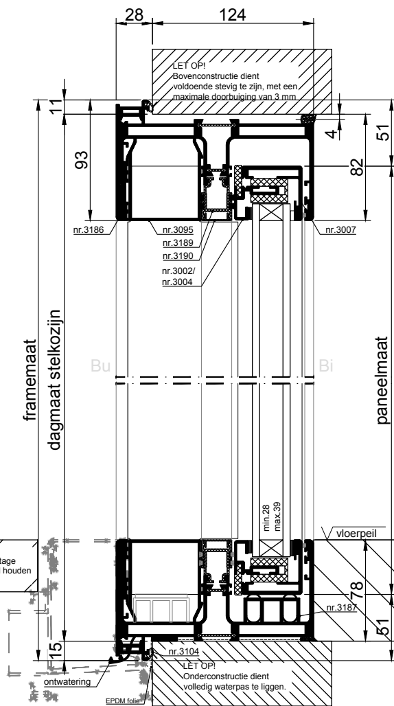
VERTECALE DOORSNEDE type XHS-10D
