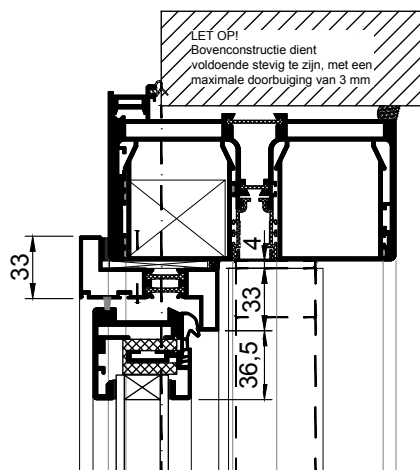
horizontaal bovenprofiel met deur
