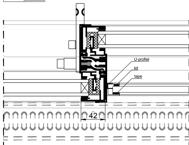
verticale middennaad met doorvalbeveiliging
