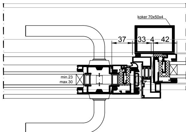
verticale tussenstijl vast paneel met deur
