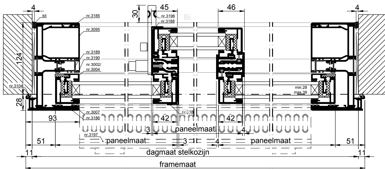
HORIZONTALE DOORSNEDE type XHS-9C
