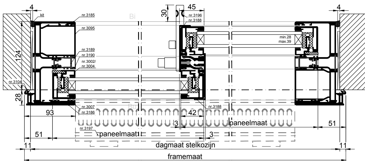
HORIZONTALE DOORSNEDE type XHS-9A
