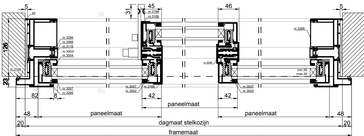
HORIZONTALE DOORSNEDE type XHS-17C
