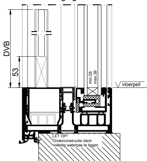
horizontaal onderprofiel met doorvalbeveiliging
