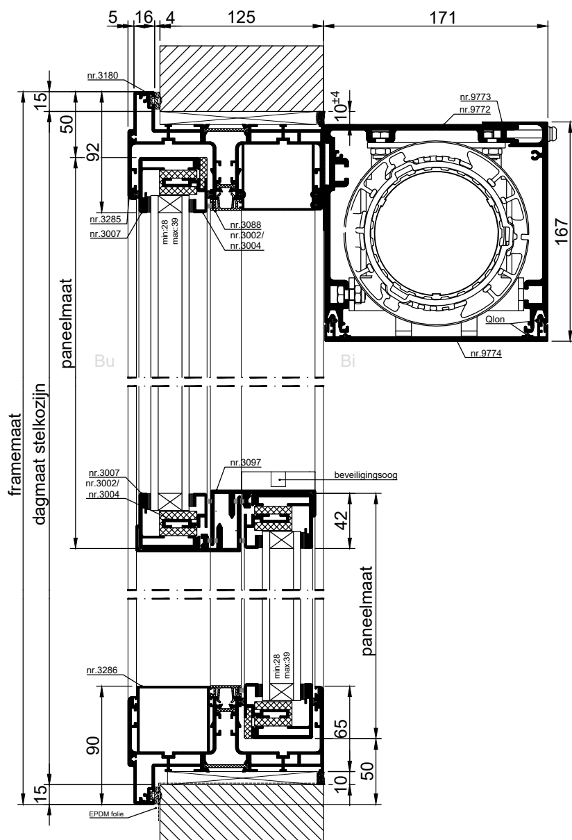
VERTICALE DOORSNEDE type XEVS-10AXL
