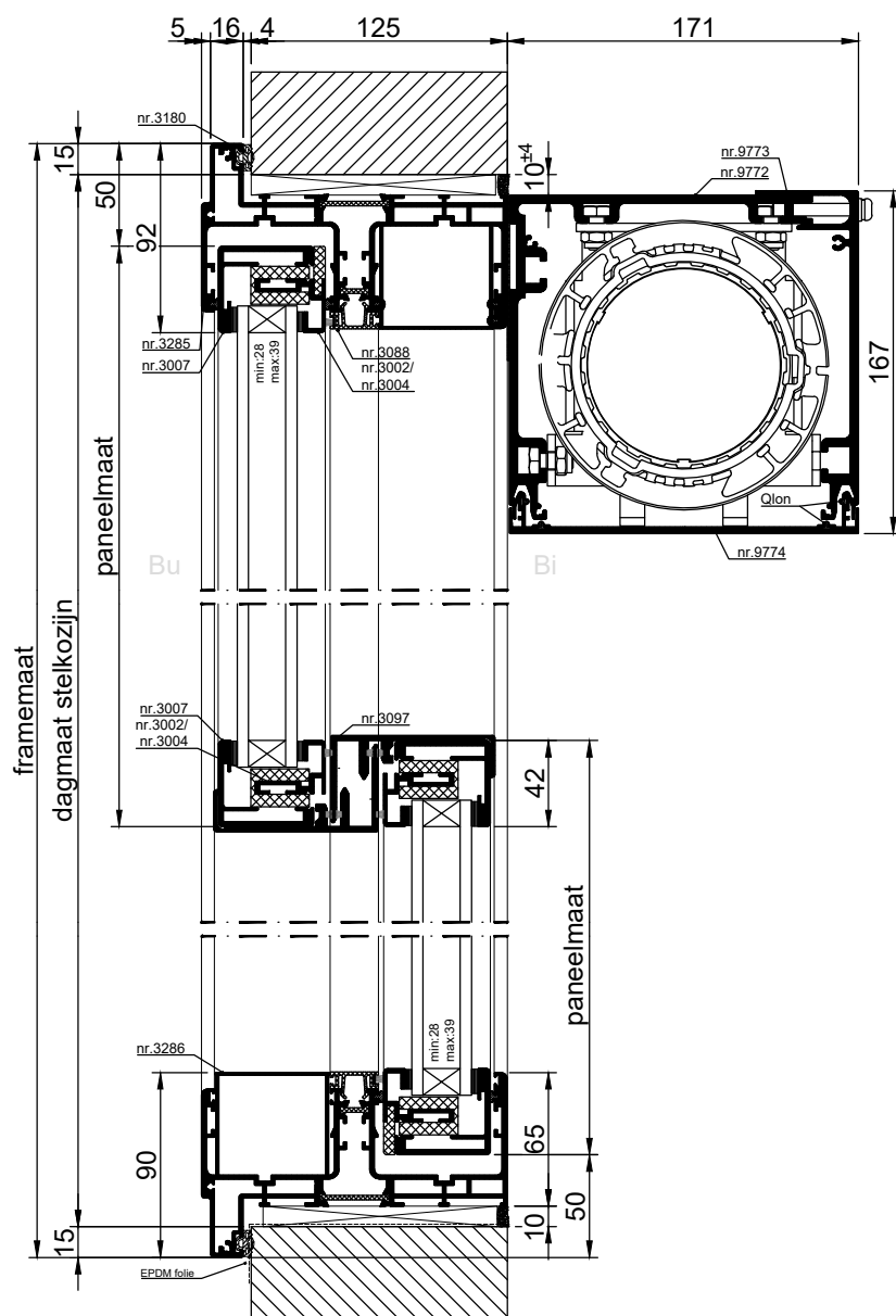
VERTICALE DOORSNEDE type XEVS-10BXL
