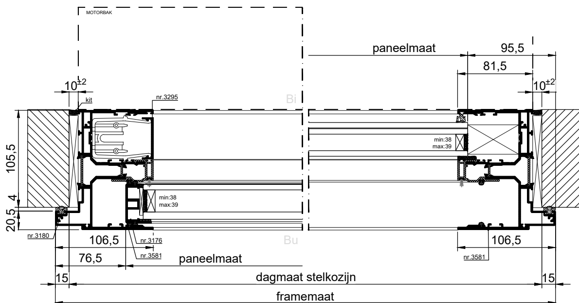
HORizontale Doorsnede type XEVS-25A
