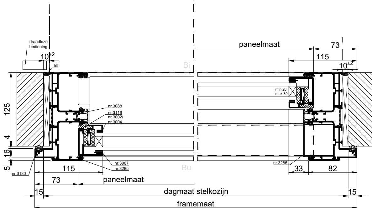
HORIZONTALE DOORSNEDE type XEVS-10BXL
