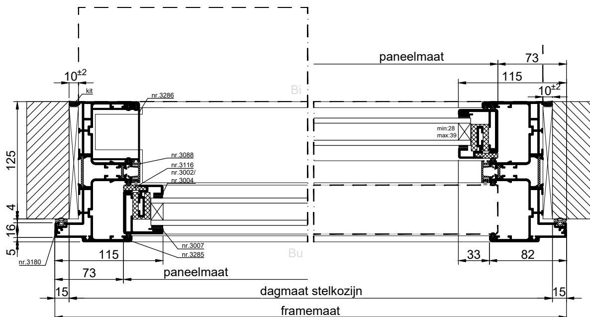
HORIZONTALE DOORSNEDE type XEVS-10A
