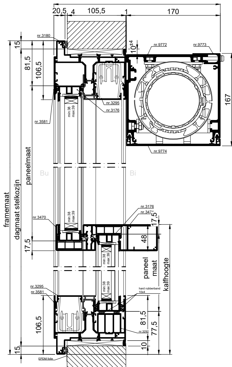
VERTICALE DOORSNEDE type XEVS-25BXL
