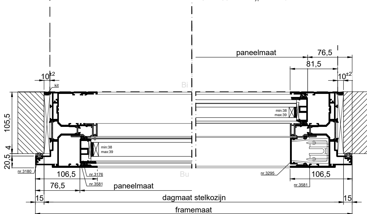
HORizontale DOORSNEDE type XEVS-25BXL
