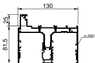
Uitvoering aanslaglip buitenzijde
