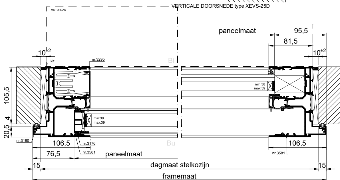
HORIZONTALE DOORSNEDE type XEVS-25D
