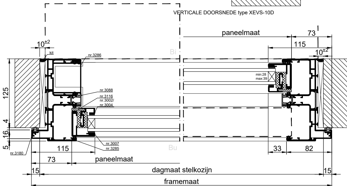
HORizontale DOORSNEDE type XEVS-10D
