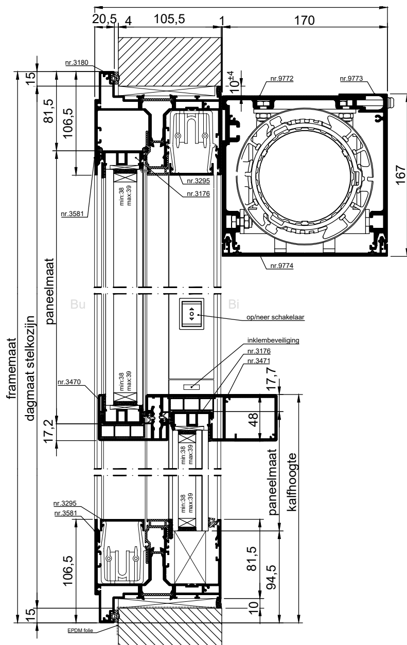
VERTICALE DOORSNEDE type XEVS-25AXL
