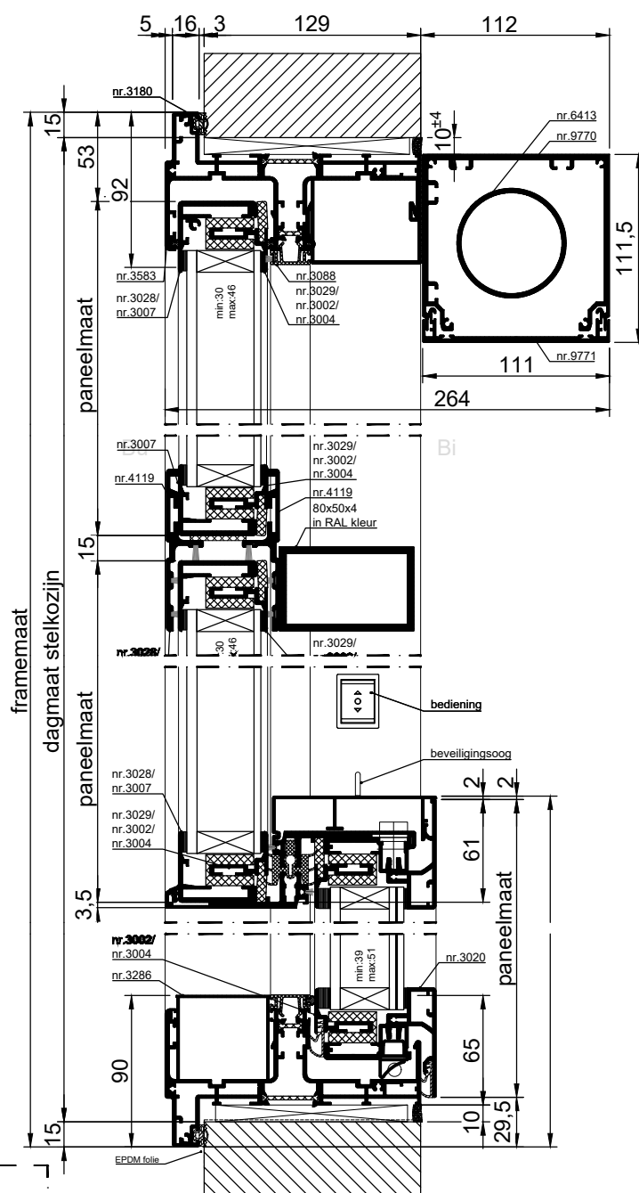
VERTICALE DOORSNEDE type XEVS-11D
