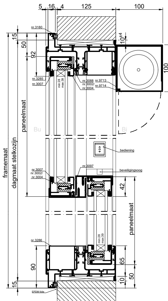
VERTICALE DOORSNEDE type XEVS-10A
