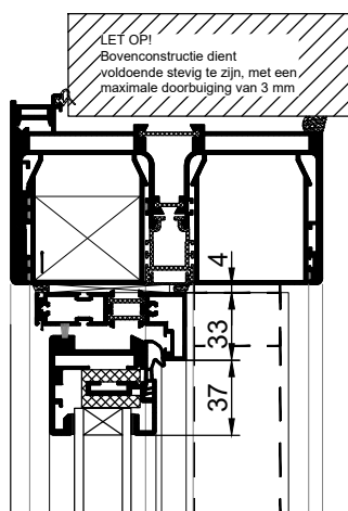
horizontaal bovenprofiel met deur
