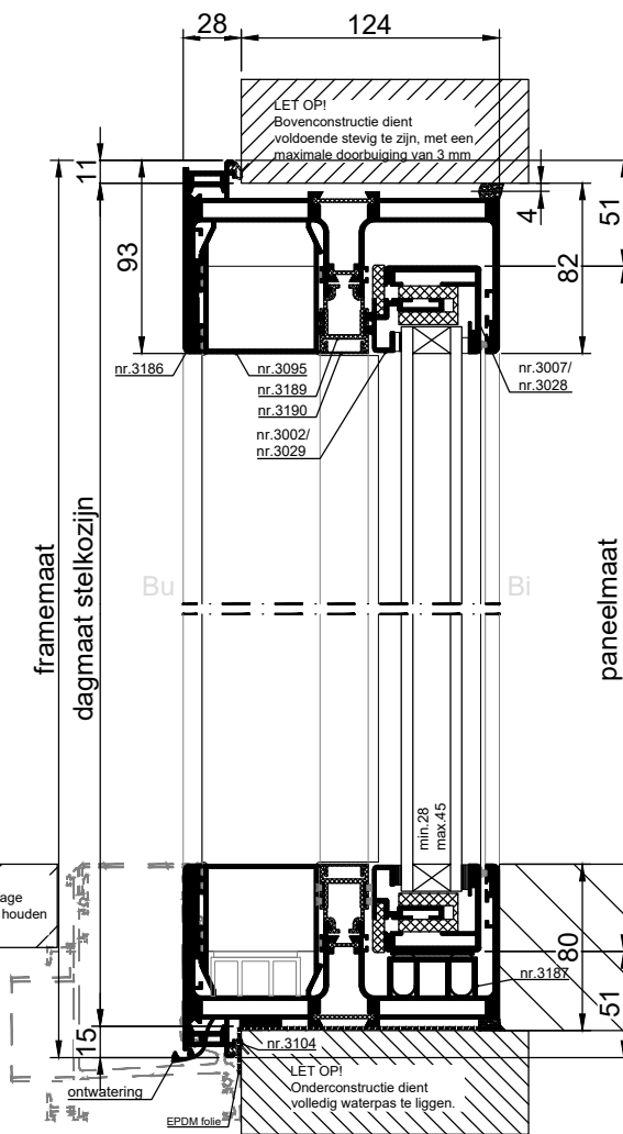
VERTICALE DOORSNEDE type XHS-9C
