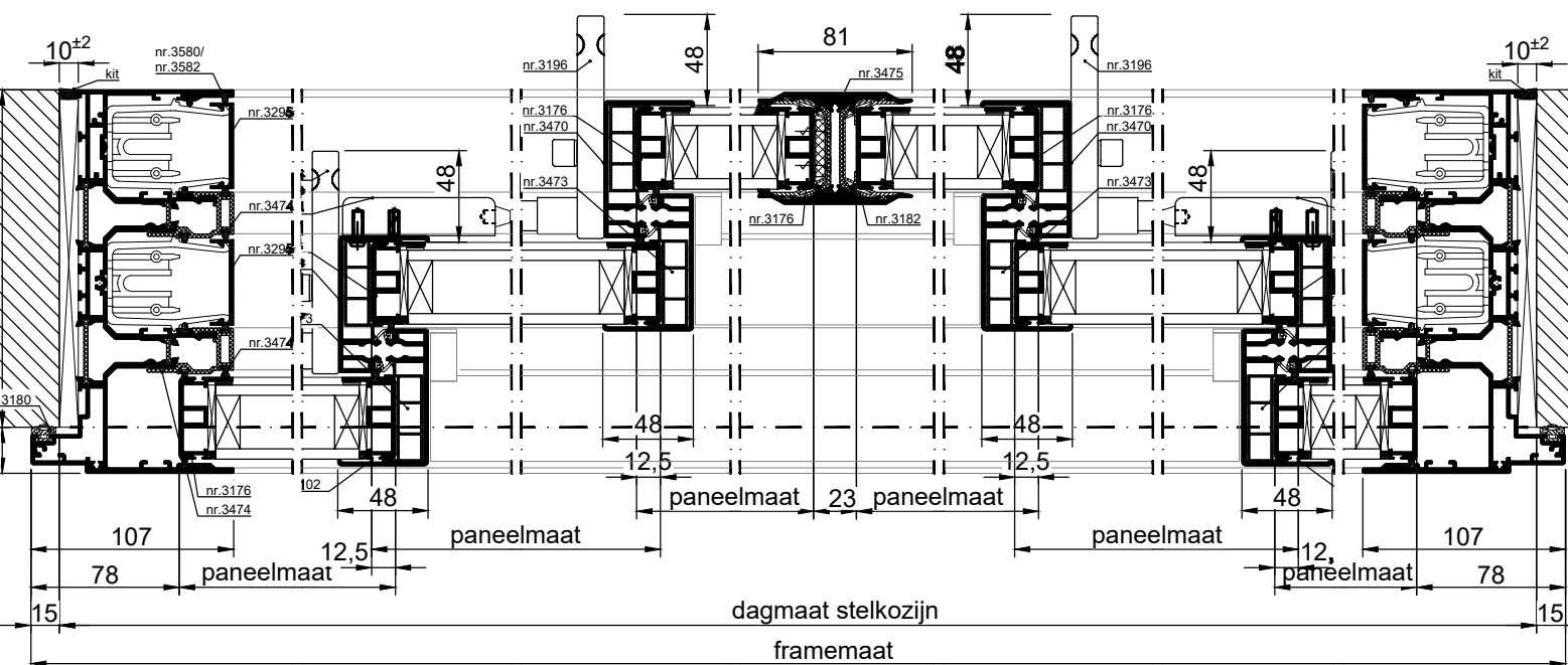
HORIZONTALE DOORSNEDE type XHS-35E
