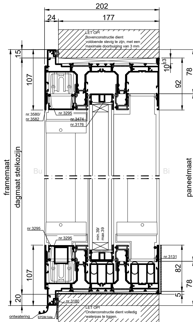
VERTICALE DOORSNEDE type XHS-35A
