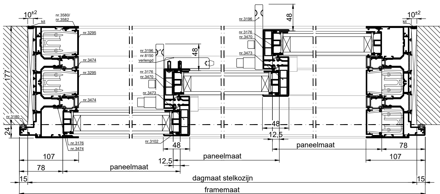
HORIZONTALE DOORSNEDE type XHS-35A
