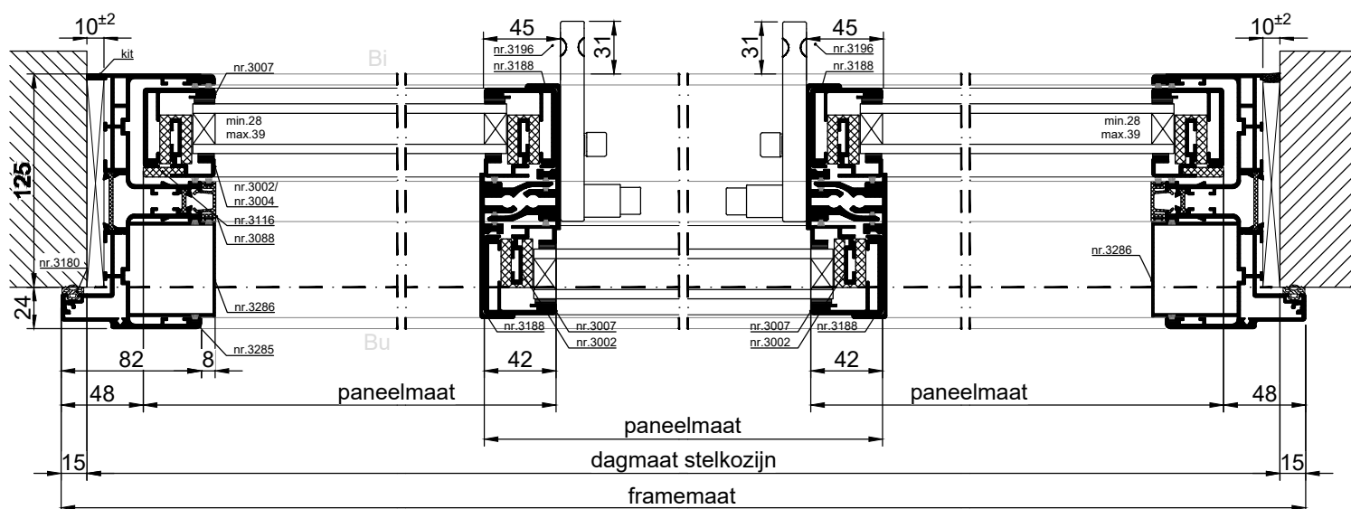
HORIZONTALE DOORSNEDE type XHS-17D
