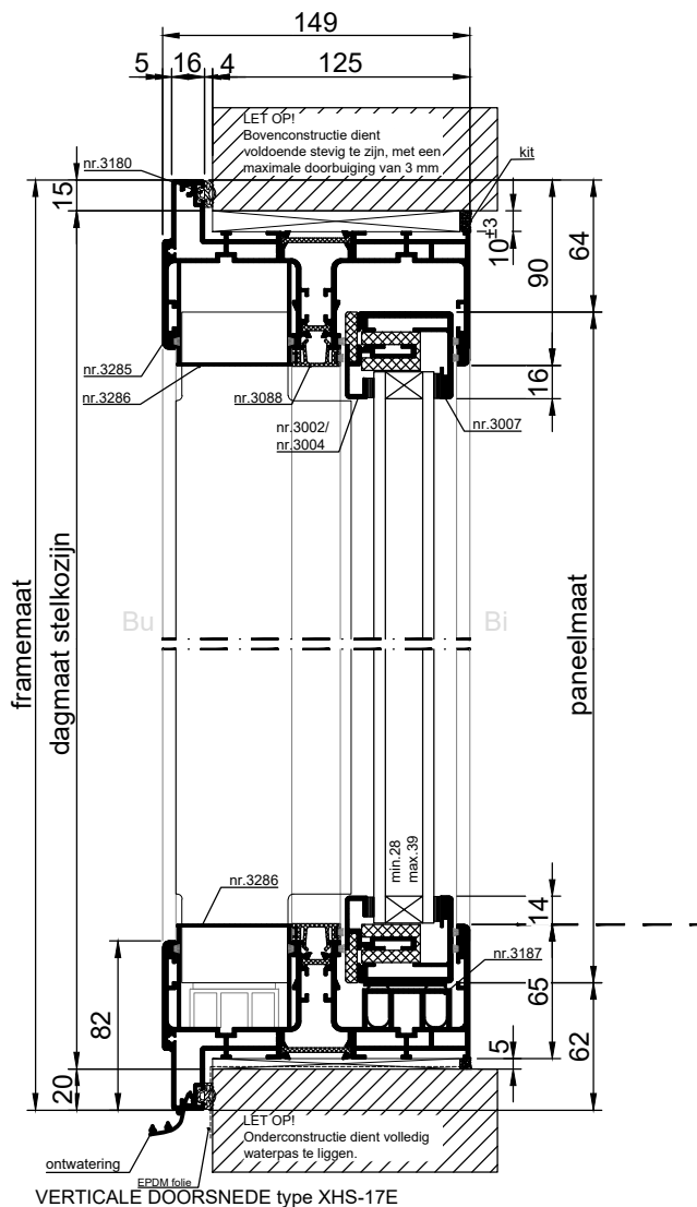
VERTICALE DOORSNEDE type XHS-17E
