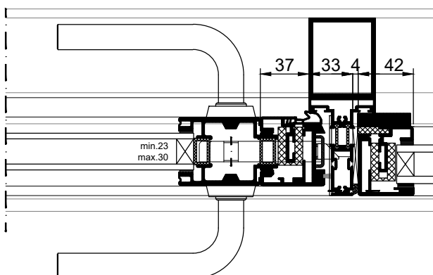
verticale tussenstijl vast paneel met deur
