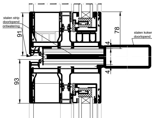
horizontale boven- en onderprofiel met koppeling
