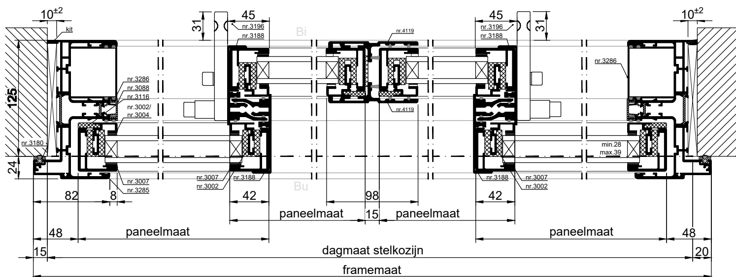
HORIZONTALE DOORSNEDE type XHS-17E
