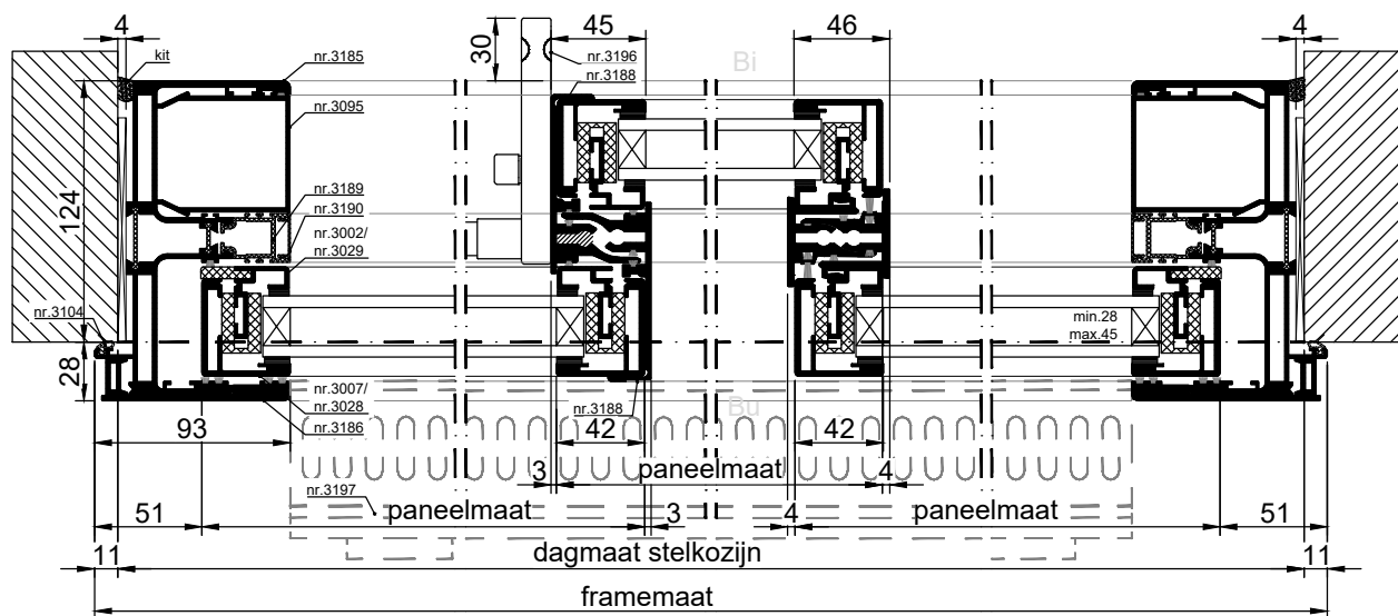
HORIZONTALE DOORSNEDE type XHS-9C
