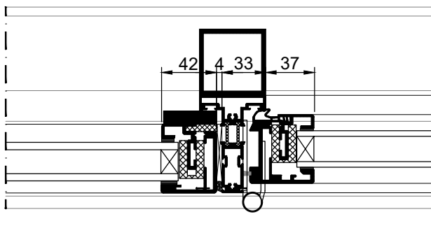
verticale tussenstijl vast paneel met deur
