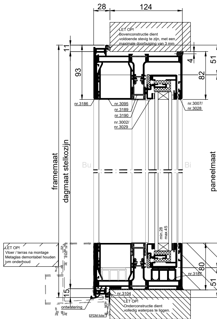
VERTICALE DOORSNEDE type XHS-9D
