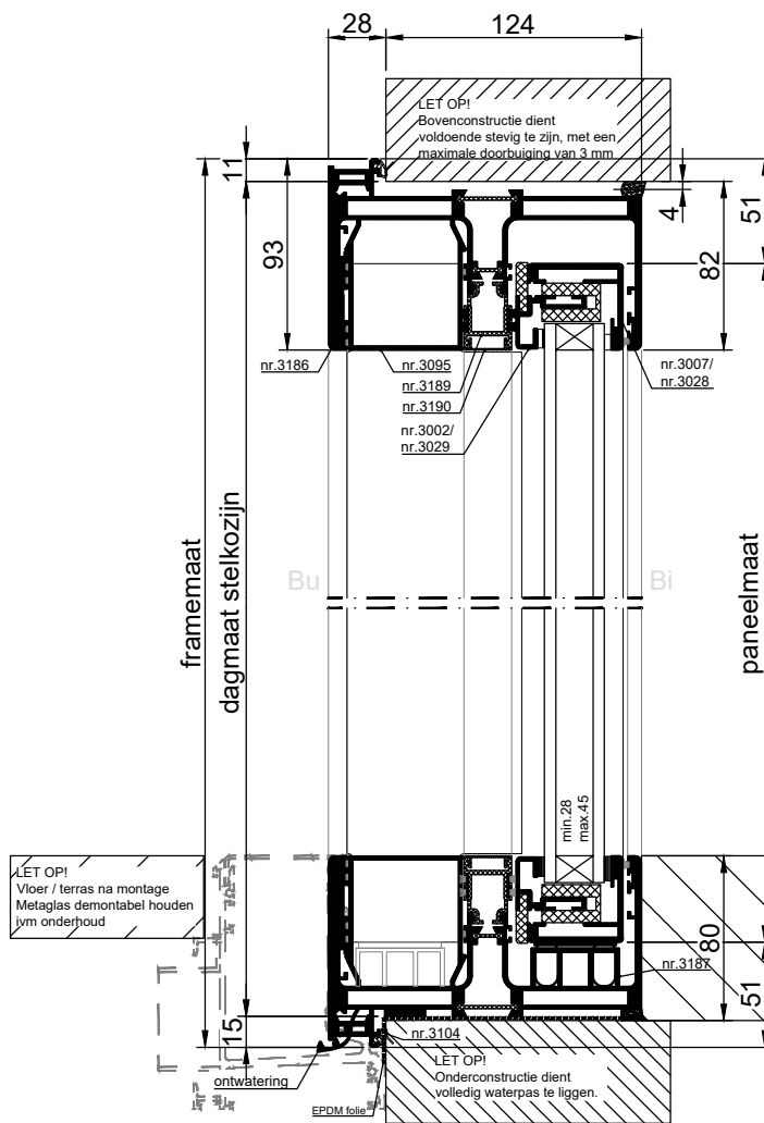
VERTICALE DOORSNEDE type XHS-10A
