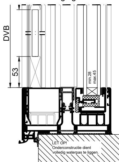
horizontaal onderprofiel met doorvalbeveiliging
