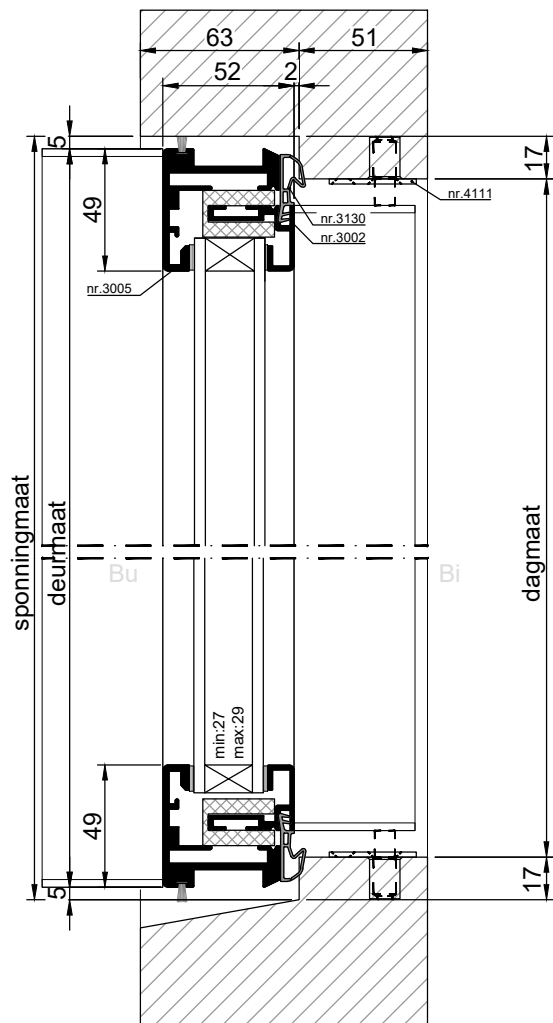
VERTICALE DOORSNEDE type MUS-6A
