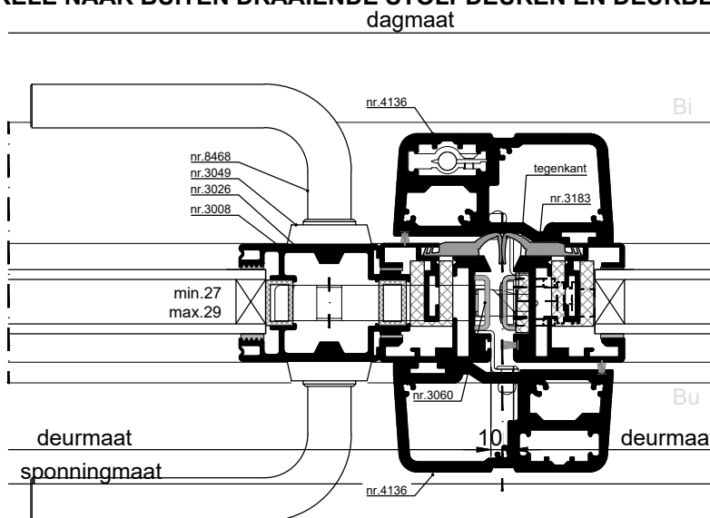
HORizontale DOORSNEDE type MUS-6A/E
