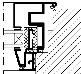
STANDAARD MONTAGE
