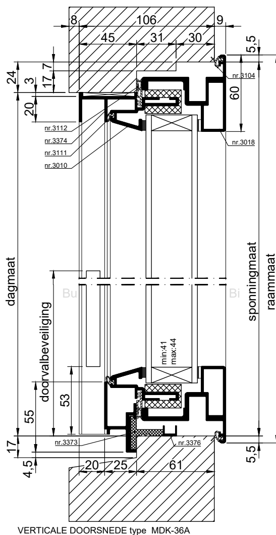
VERTICALE DOORSNEDE type MDK-36A
