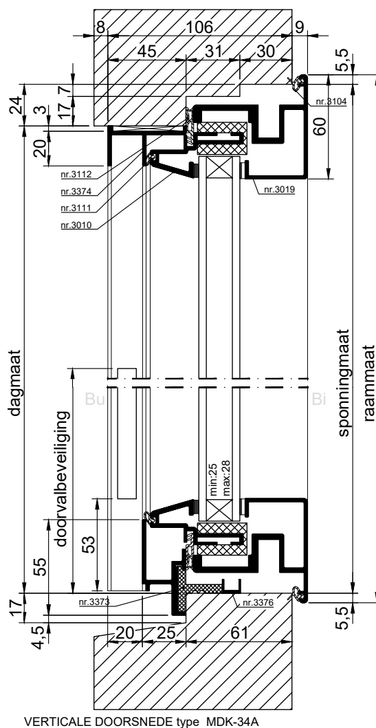
VERTICALE DOORSNEDE type MDK-34A
