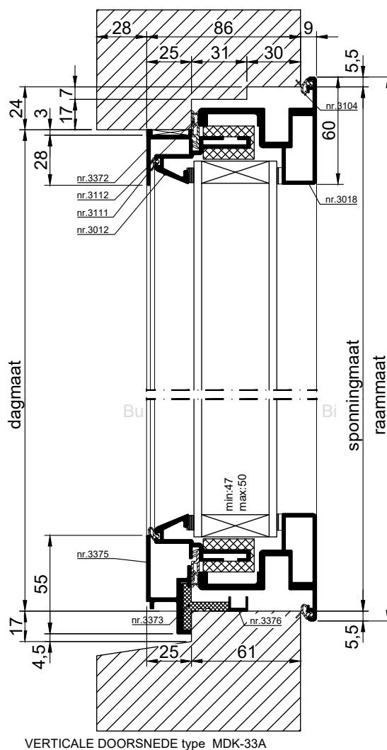
VERTICALE DOORSNEDE type MDK-33A
