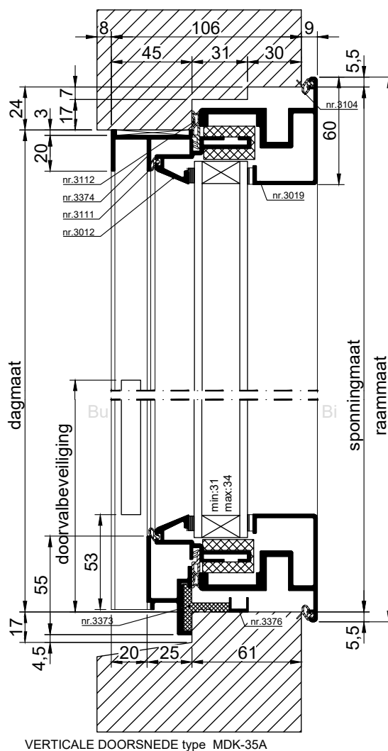
VERTICALE DOORSNEDE type MDK-35A
