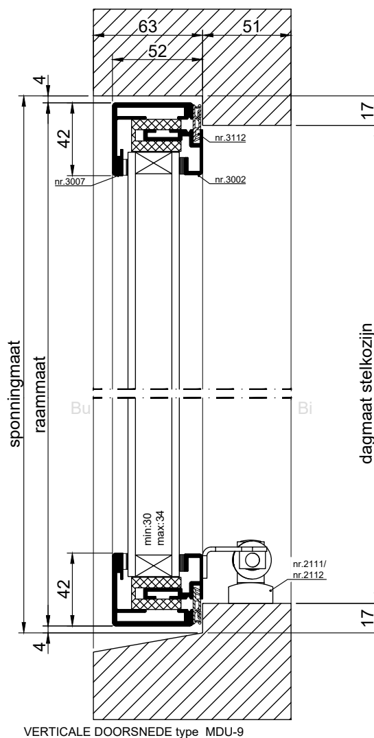
VERTICALE DOORSNEDE type MDU-9
