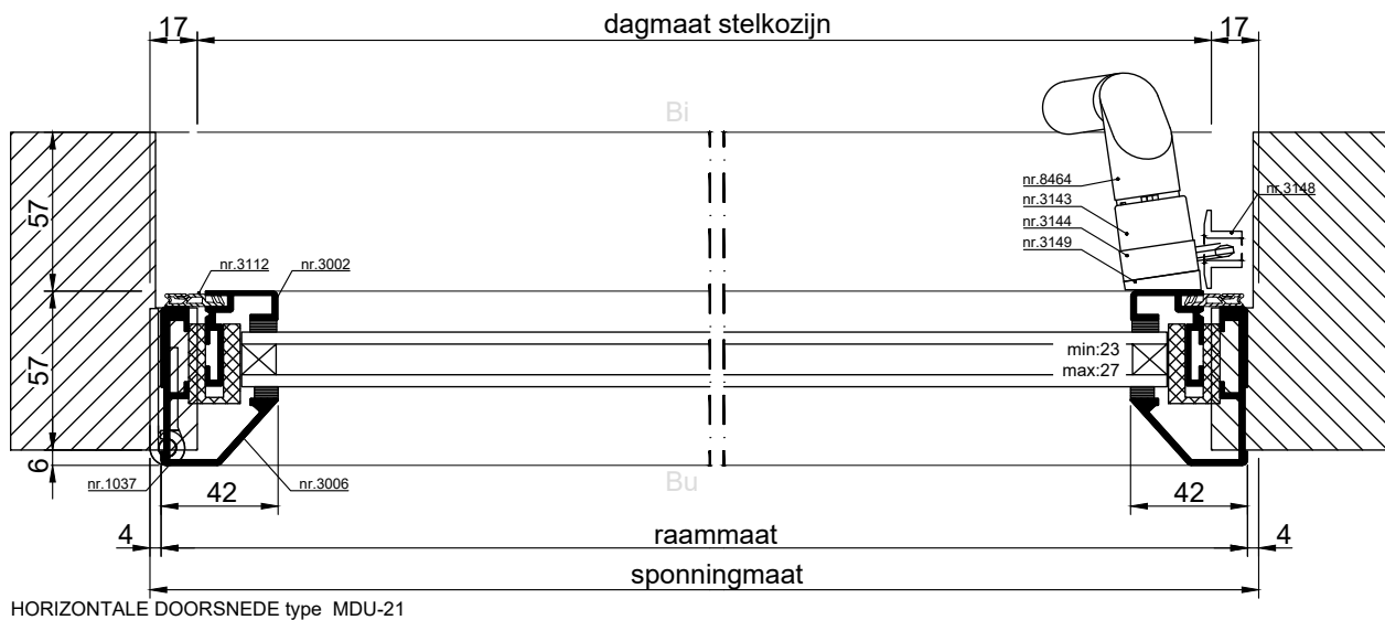
HORIZONTALE DOORSNEDE type MDU-21
