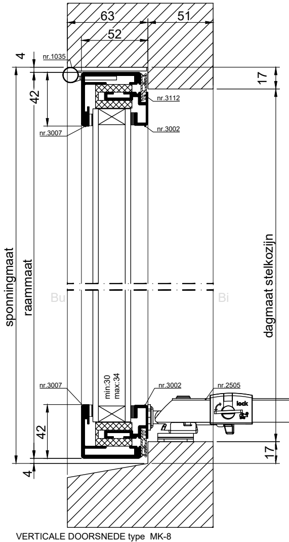
VERTICALE DOORSNEDE type MK-8
